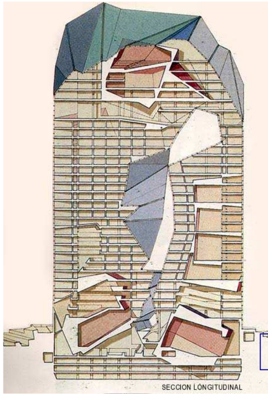
SECCION LONGITUDINAL
