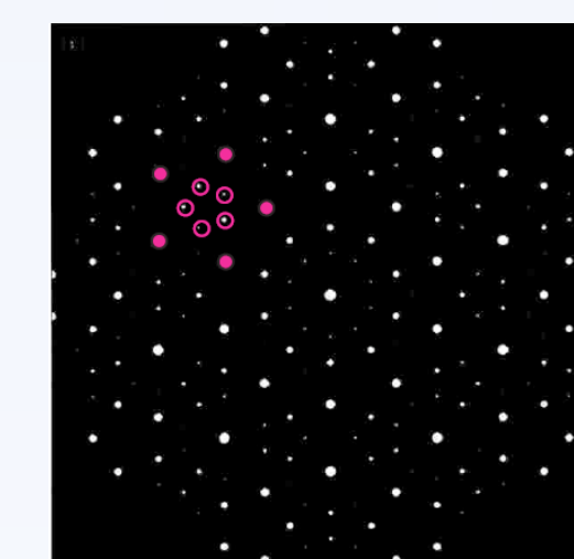
Patrón de difracción para casi-cristal: se muestran en blanco los puntos de mayor intensidad. Se encuentran marcados en rojo algunos pentágonos de este patrón.
