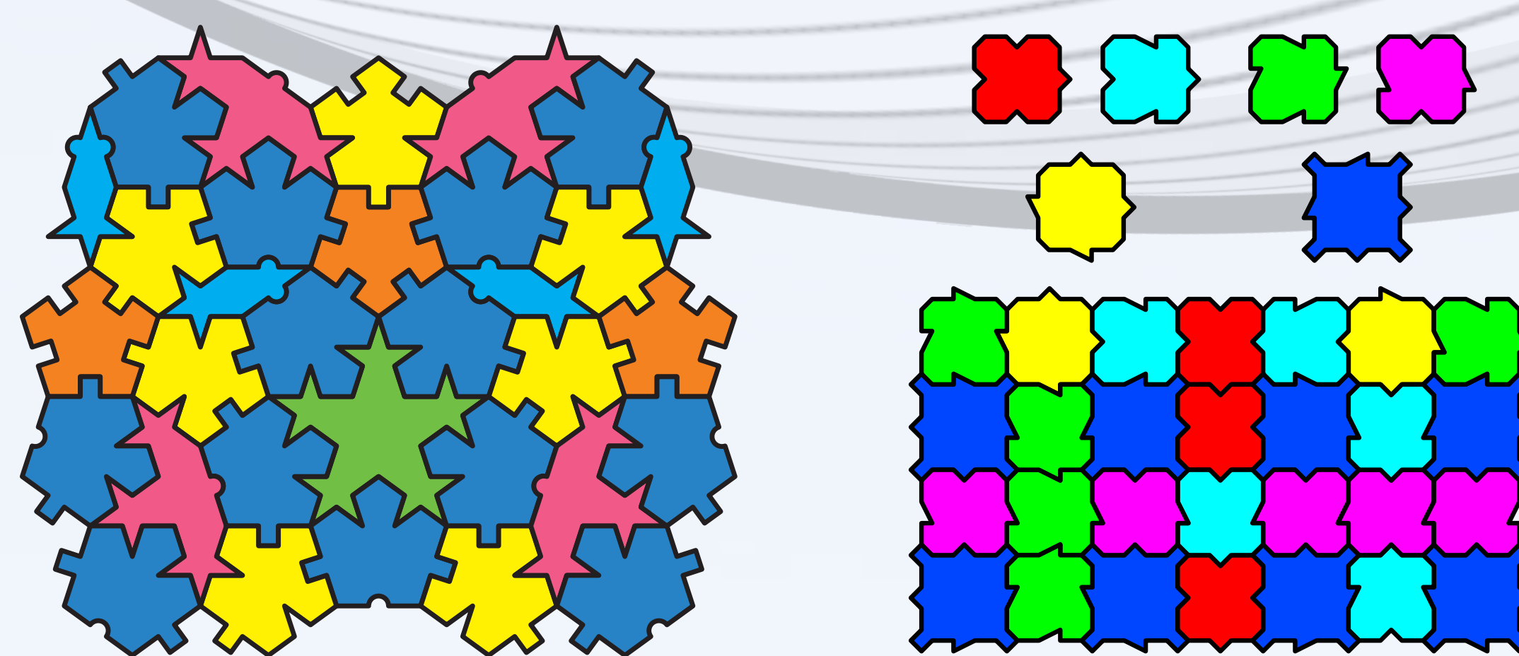
Motivos en los mosaicos aperiódicos y repetitivos de Penrose y Robinson respectivamente.
