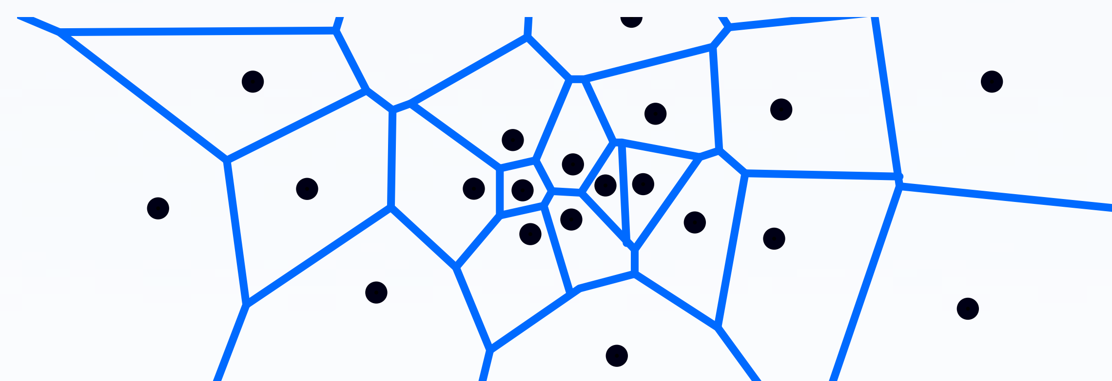
Un conjunto de Delone es un conjunto D en el que los puntos distan más que una cierta distancia r , pero que dado un punto cualquiera del plano, es posible encontrar uno de D a distancia menor que una cierta cantidad R .
