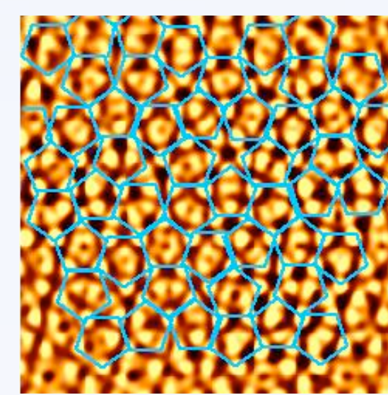
La estructura molecular interna de un casi-cristal, que produce un mosaico del plano con simetría pentagonal. El mosaico de Penrose se ha superpuesto en azul.
