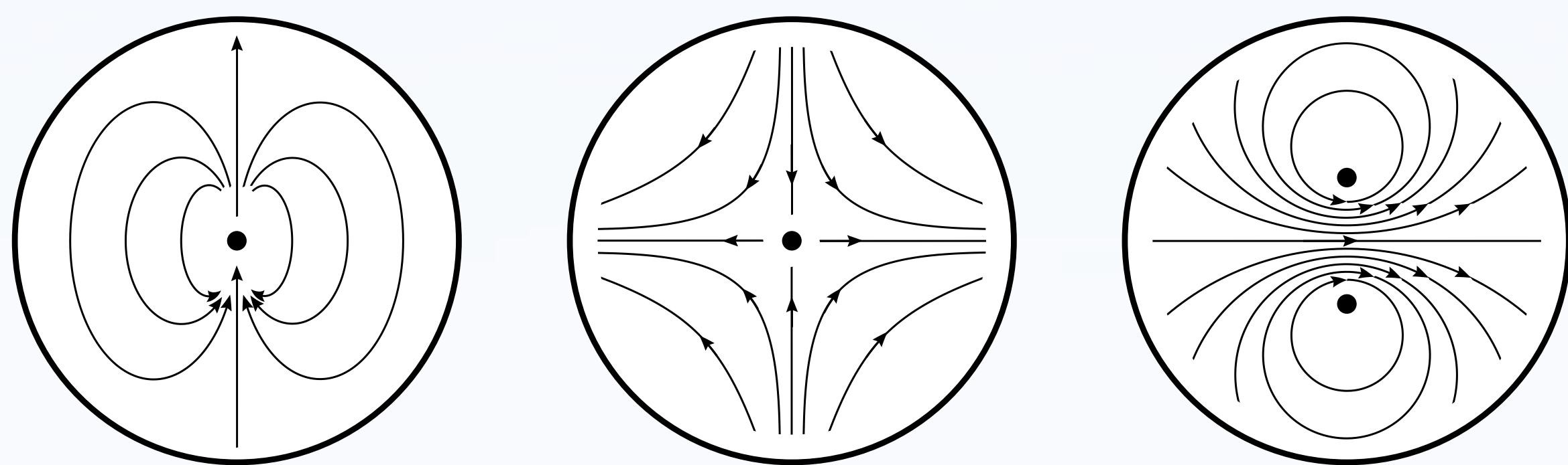
Campos de vectores en el plano con singularidades.
