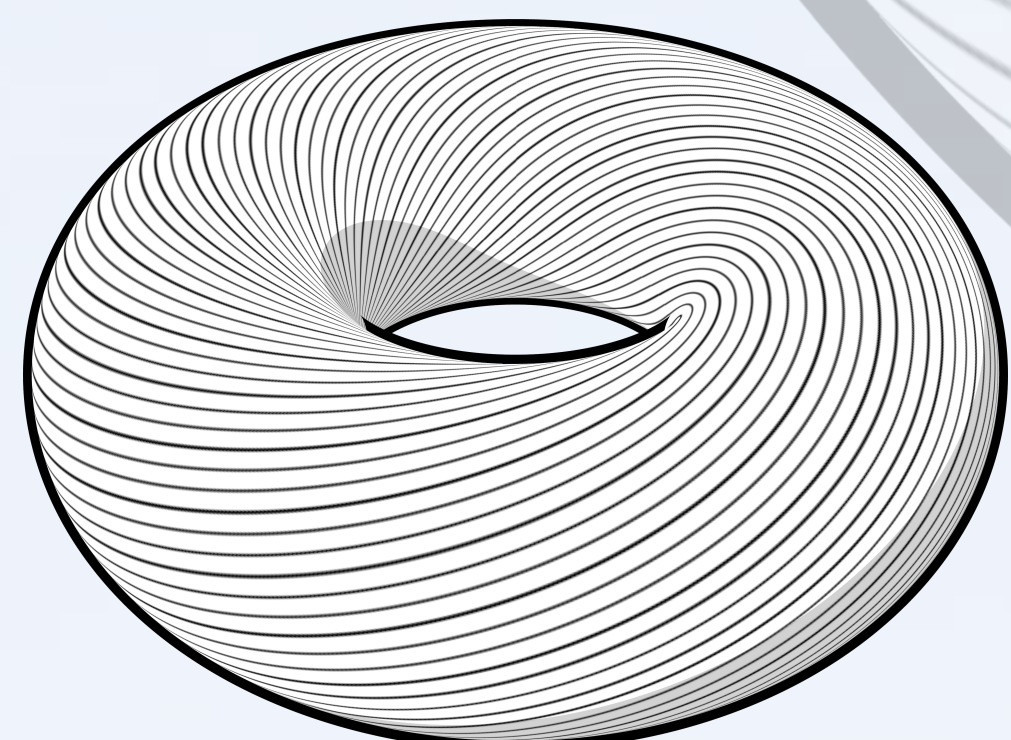
Las rectas de una misma pendiente irracional fija inducen una foliación del toro T^2 por rectas que se enrollan indefinidamente.
